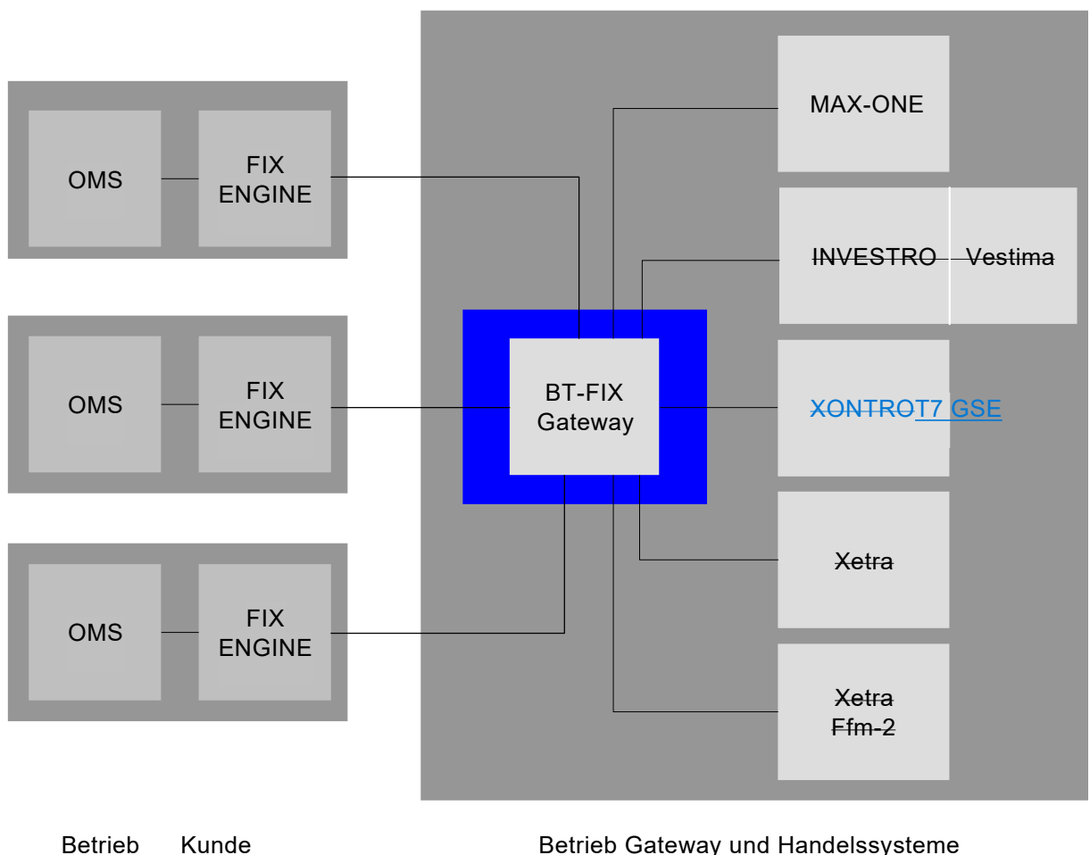
Abbildung 1-1: Systemüberblick
